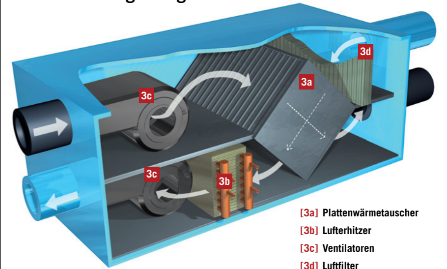
Detail Lüftungsanlage
