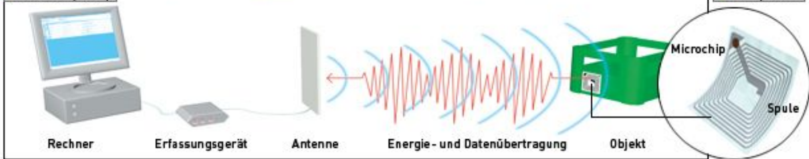
1 Funktionsprinzip
